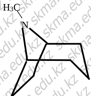
Тропин
