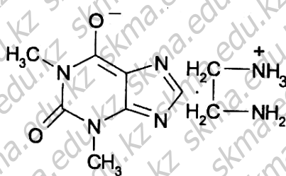
Эуфиллин – Euphillinum.
