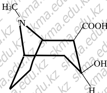
Эггонин
