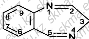
3H-1,4-Бензодиазепин
