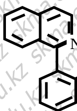
Бензилизохинолин
