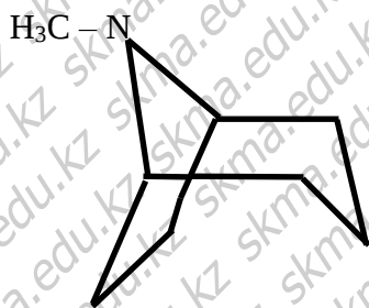
Тропан
