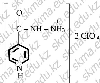
Изониазидтің дихлораты
