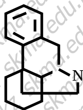
Морфинан
