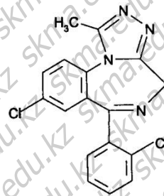
Триазолам 8-Хлор-6-(2-хлорфенил)-1-метил-4Н-[1,2,4]триазоло[4,3а]-1,4-бензодиазепин
