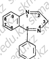
5-Фенил-3Н-1,4-бензодиазепин
