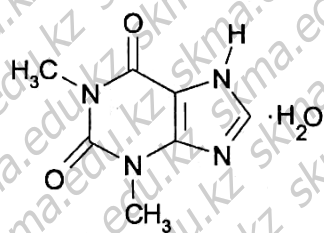
Теofilлин-Theophyllinum. 1,3-Диметилксантин.
