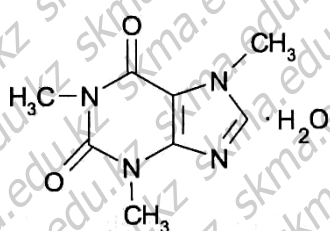
Кофеин-Coffeinum. 1,3,7-Триметилксантин.
