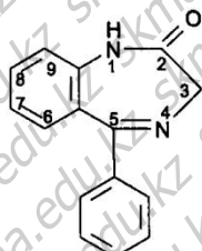
1,2-Дигидро-3Н-1,4-бензодиазепин-2-он
