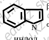
индол
