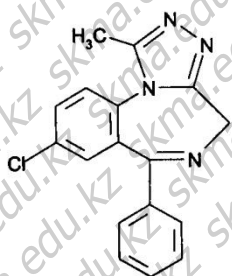
Алпрозолам 8-Хлор-1-метил-6-фенил-4Н-[1,2,4]триазоло[4,3а]-1,4-бензодиазепин
